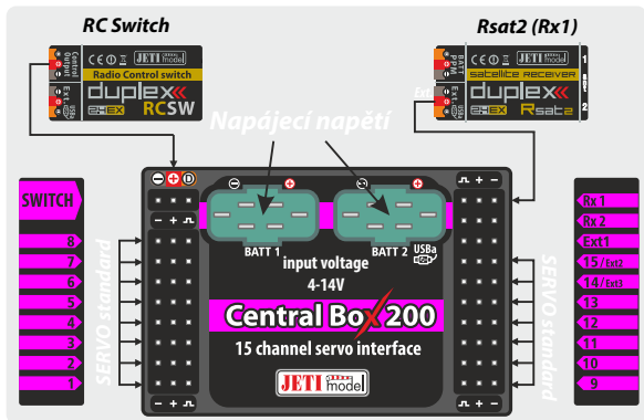
Obr. 4: Aplicační zapojení s RC Switchem
