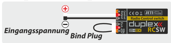
Bild. 1: Binden des RC Switch
