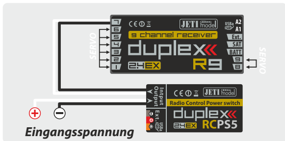
Bild 5: Anschluss Beispiel mit RC Power Switch
