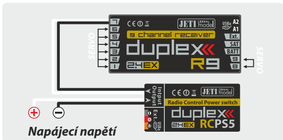
Obr. 5: Aplicační zapojení s RC Power Switchem
