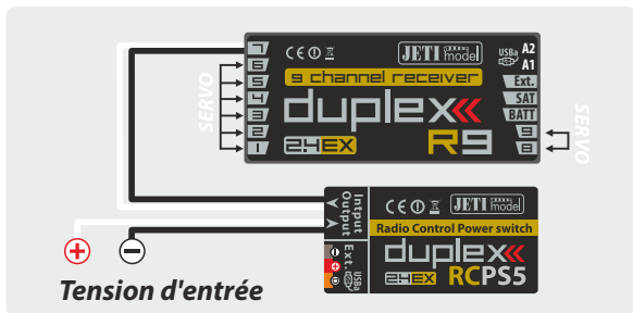
Fig. 5: Exemple de connexion avec RC Power Switch
