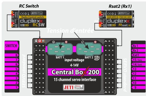
Fig. 4: Exemple de connexion avec RC Switch
